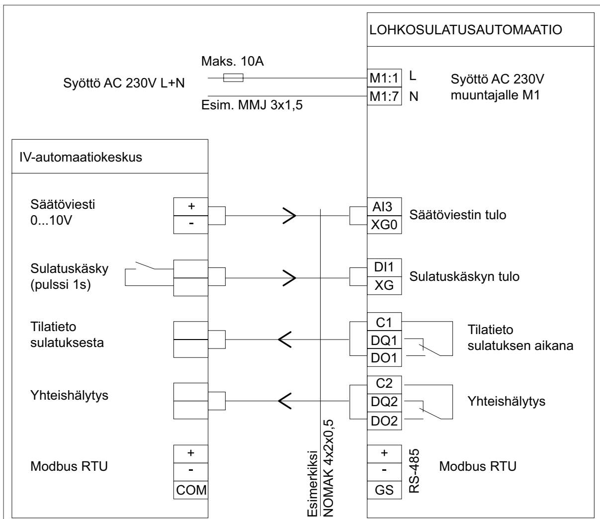
Lohkosulatusautomaation sähkönsyöttö
