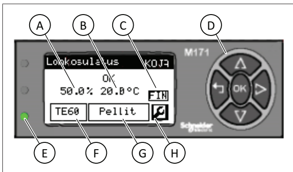
Ohjauspaneeli
